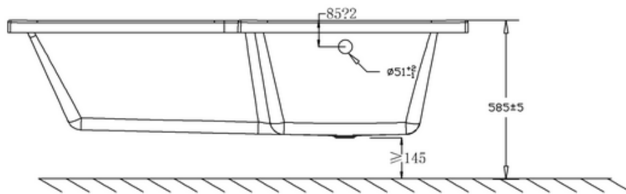
A-A
