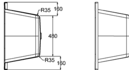
B-B
