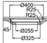
C SCALE 1:2
